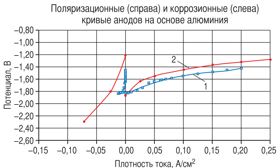
Рис. 20. Высокоэффективные аноды, используемые в качестве топлива в воздушно-алюминиевых топливных элементах: 1 – разработанные в ОИВТ РАН; 2 – используемые фирмой Altek fuel group, Inc (США)
