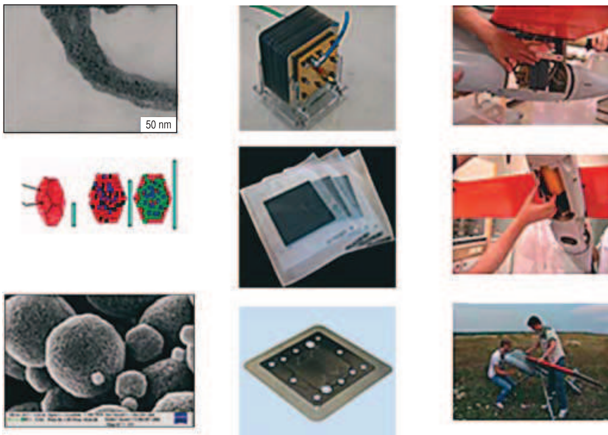
Топливный элемент и его компоненты: а) ТЭ в сборке, б) мембранно-электродный блок, в) биполярная пластина
